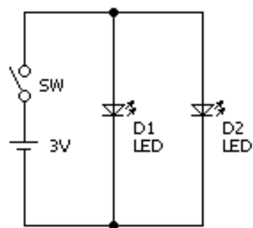
図3 警告灯の回路図
